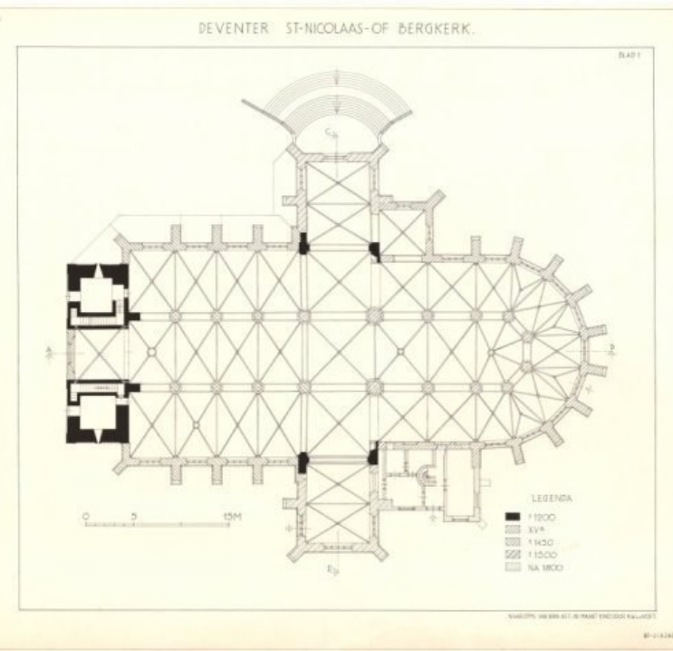
Plattegrond van de Bergkerk van architect te Riele uit het begin van de 20e eeuw.
